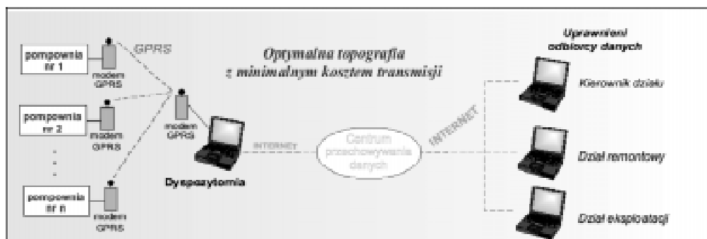
Monitoring przepompowni ścieków przez Internet z wykorzystaniem GPRS
