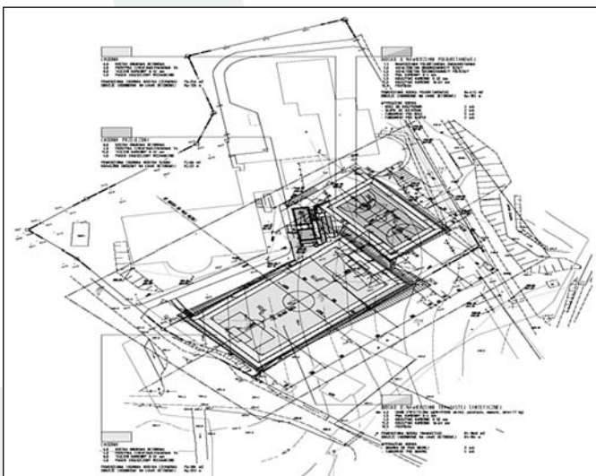
Projekt zagospodarowania terenu przy Gimnazjum w Istebnej.
